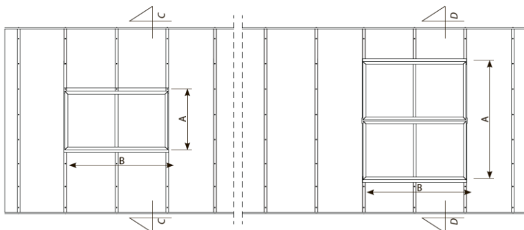
Рисунок 3. Поперечные сечения стандартной конструкции арочной световой полосы со встроенными люками
