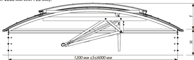
Поперечное сечение C-C арочной световой полосы с односторчатым люком для дымоудаления и вентиляции
